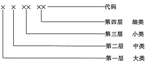
图 1 代码结构
